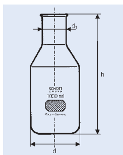
Flacons pour milieux de culture à bord évasé
