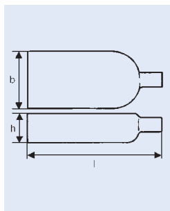
Ballon à culture selon Roux col conique, excentrique
