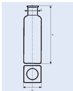
Flacons carrés selon Breed-Demeter
